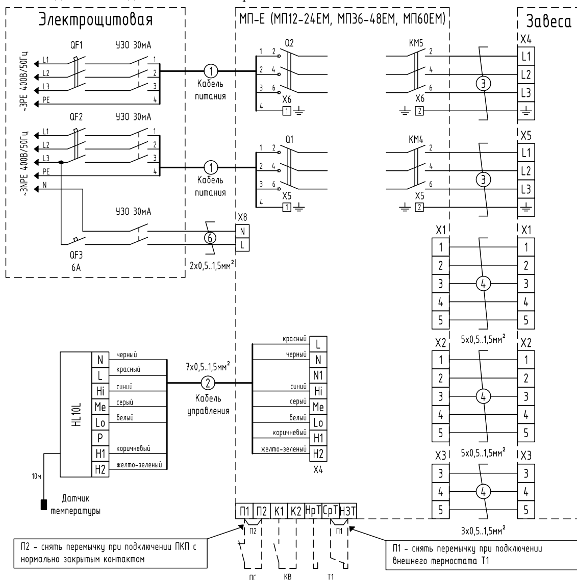
Рисунок 1. Схема подключения одной завесы к электрической сети
