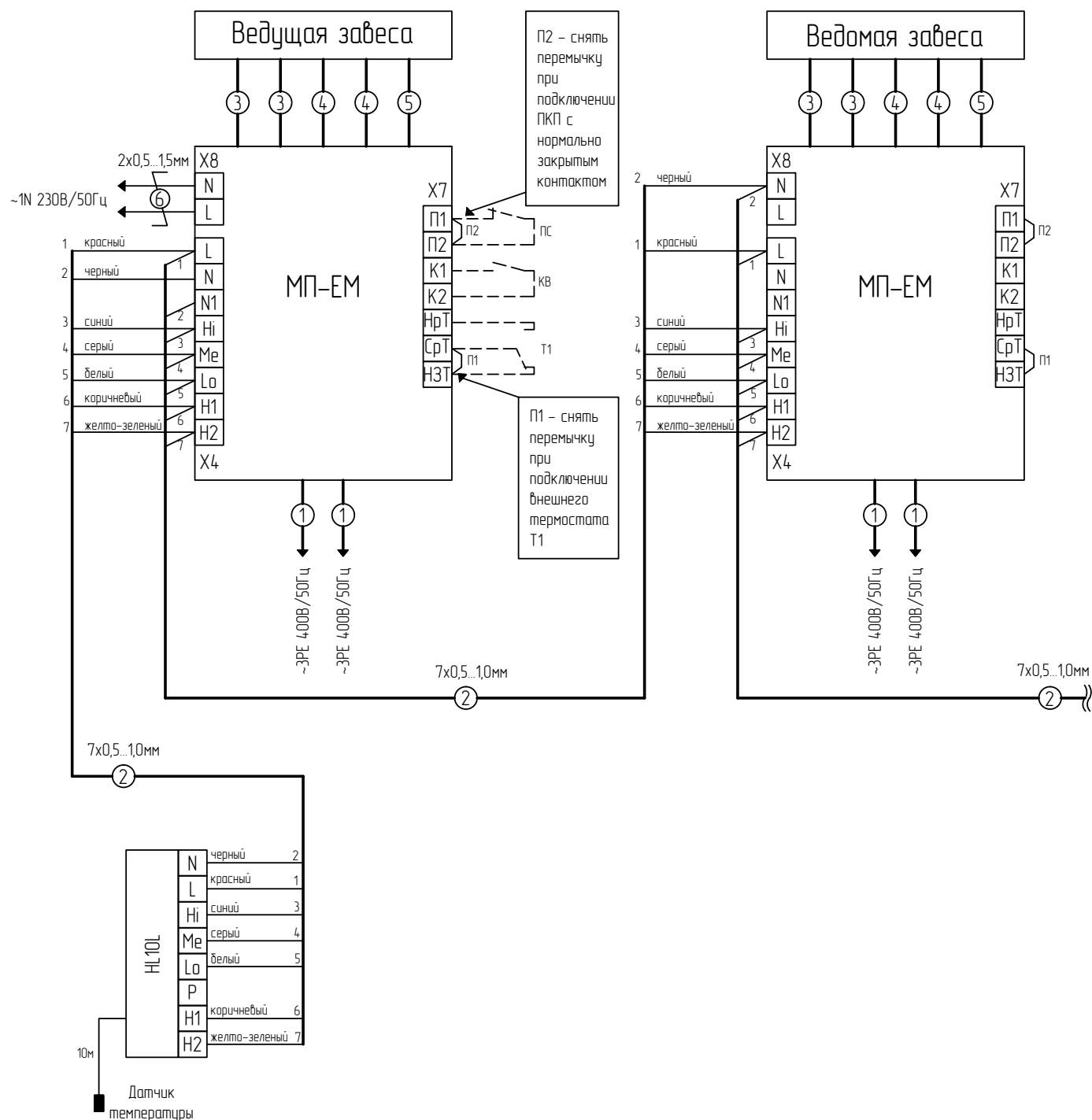
Рисунок 2. Схема подключения группы от двух до двадцати завес к одному пульту управления HL10L
